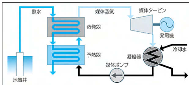
(図)バイナリー方式の仕組み ※地下に掘削した井戸の深さは1,000～3,000m
